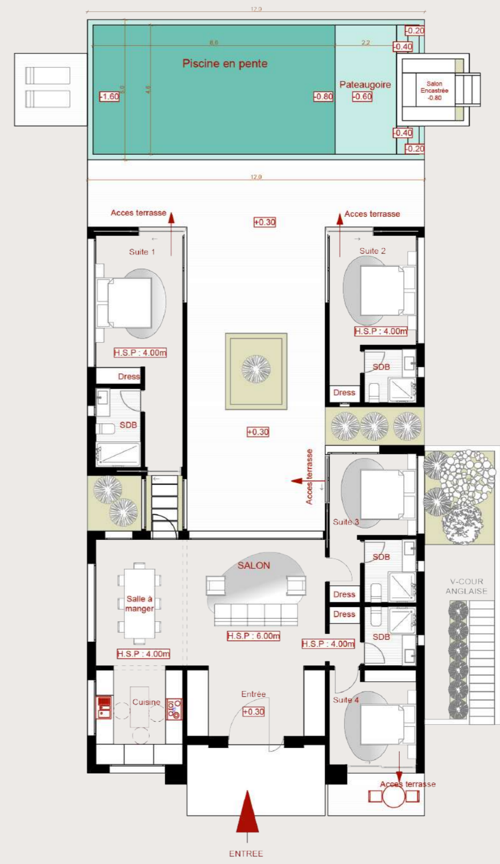
Plan d'architecte rez de chaussée
