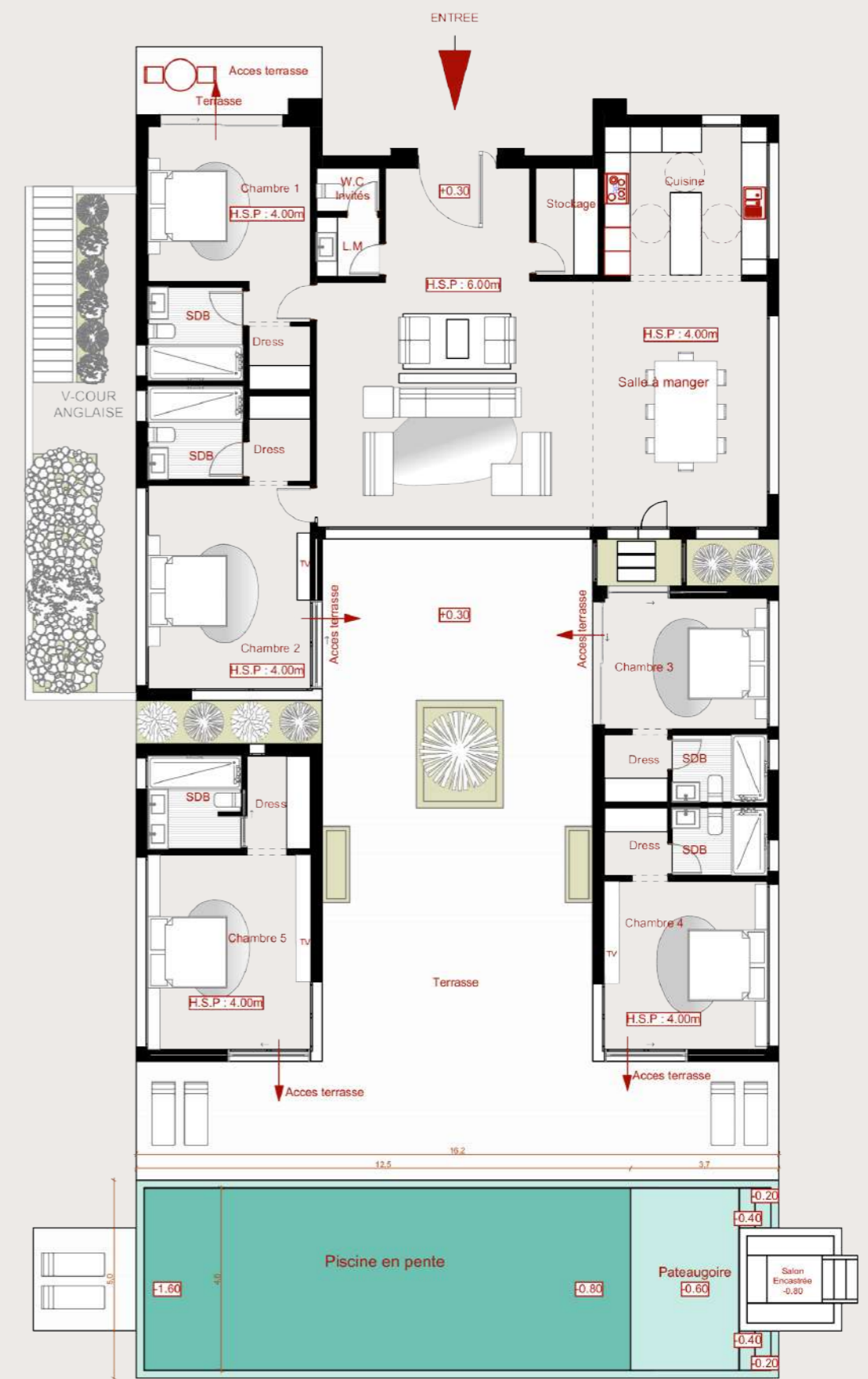
Plan d'architecte rez de chaussée
